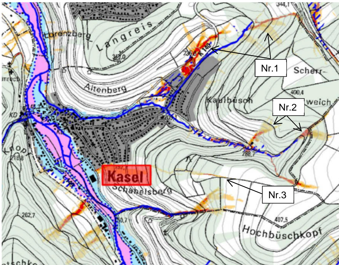
ABBILDUNG 8: KARTE „GEFÄHRDUNGSANALYSE STURZFLUT NACH STARKREGEN“ DES LFU MIT EINEM AUSSCHNITT DER ORTSGEMEINDE KASEL MIT NUMMIERUNG DER STANDORTE DER HOHEN ABFLUSSKONZENTRATIONEN (QUELLE: LFU)
