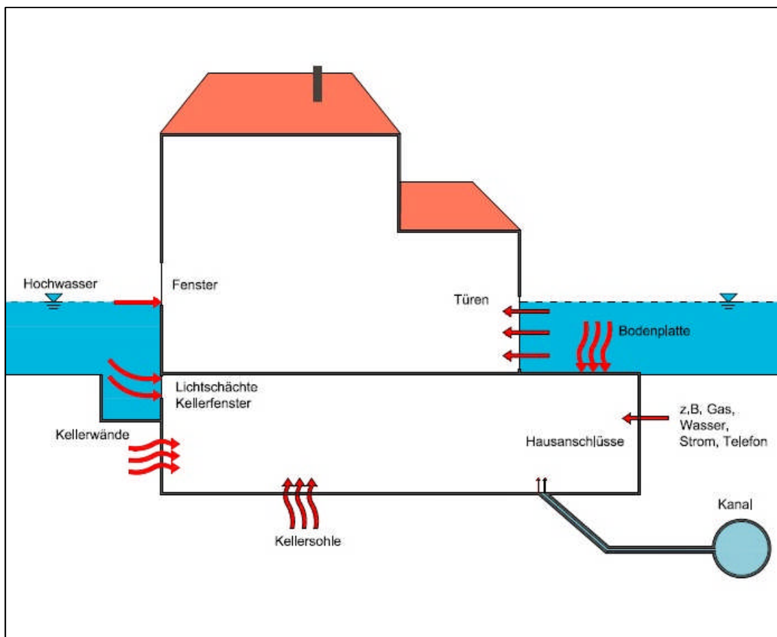
ABBILDUNG 12: EINDRINGPFADE INS GEBÄUDE [KOMPETENZZENTRUM FÜR HOCHWASSERMANAGEMENT UND BAUVORSORGE, 2015]
