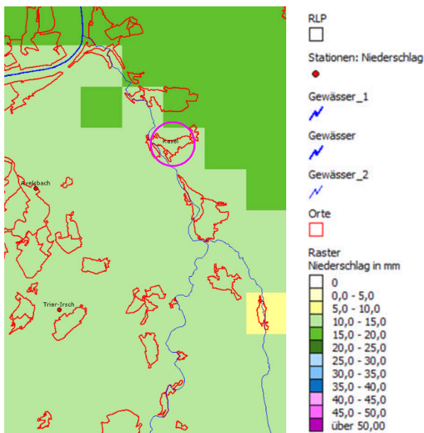
ABBILDUNG 3: GRAFISCHE ÜBERSICHT DER ÖRTLICHEN NIEDERSCHLAGSVERHÄLTNISSE VOM 05.07.2012 UM KASEL (INTERMET, QUELLE: LFU 25.10.2022)
