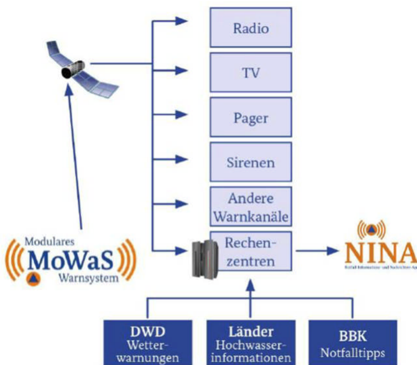
ABBILDUNG 19: MODULARES WARNSYSTEM MOWAS (BUNDESAMT FÜR BEVÖLKERUNGSSCHUTZ UND KATASTROPHENHILFE)
