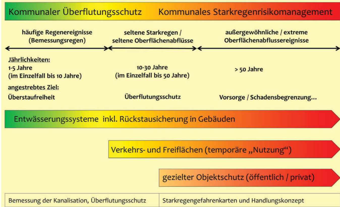
ABBILDUNG 31: ABGRENZUNG KOMMUNALER ÜBERFLUTUNGSSCHUTZ – KOMMUNALES STARKREGENRISIKOMANAGEMENT (LANDESANSTALT FÜR UMWELT, MESSUNGEN UND NATURSCHUTZ BADEN-WÜRTTEMBERG (LUBW), 2016)
